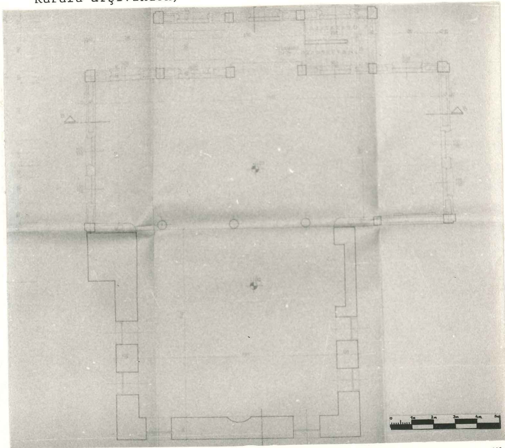
RESİM 46- Kethüda cami, üst kat restorasyon planı (G.E.E.Anıtlar Yüksek Kurulu arşivinden)
