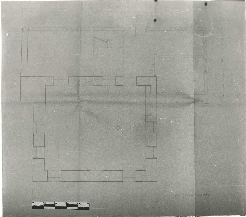
RESİM 43- Kethüda cami, alt kat rölöve planı (G.E.E.Anıtlar Yüksek Kurulu arşivinden)
