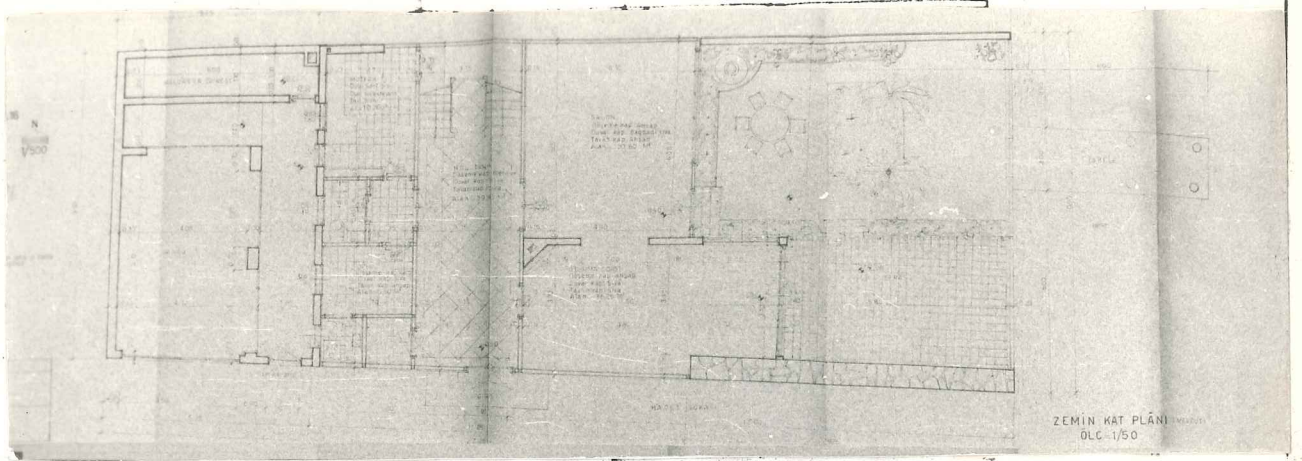
RESİM 61- Alfred Riddle Yalısı, zemin kat planı (G.E.E. ve Anıtlar Yüksek Kurulu arşivi)
