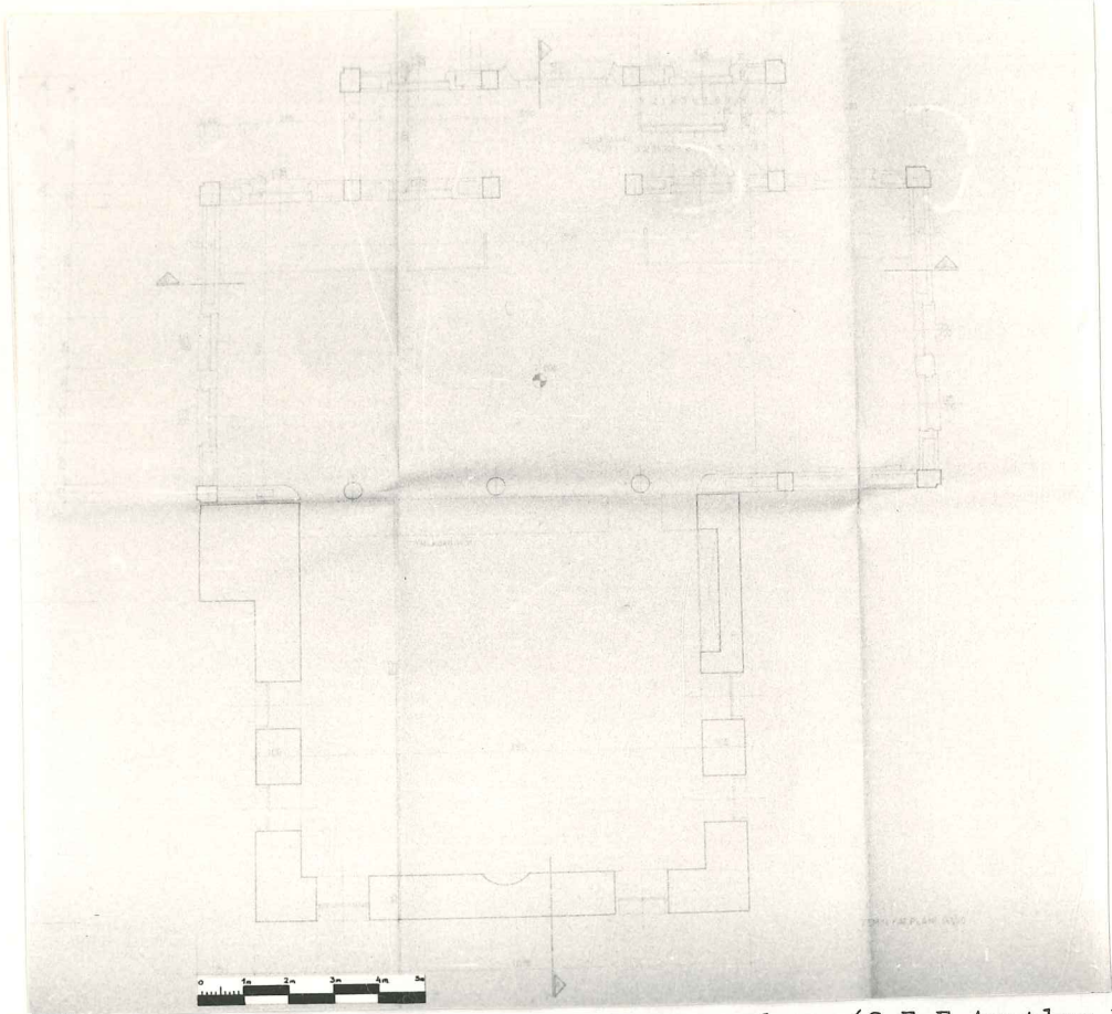
RESİM 45- Kethüda cami, Zemin kat restorasyon planı (G.E.E.Anıtlar Yüksek Kurulu arşivinden)
