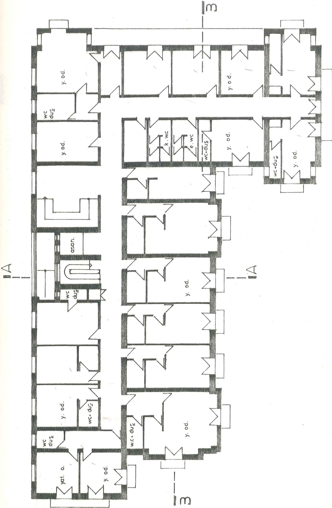
RESİM 29- Anadolu Kulübü, Otel Binası. 1. Kat Planı 1/200
