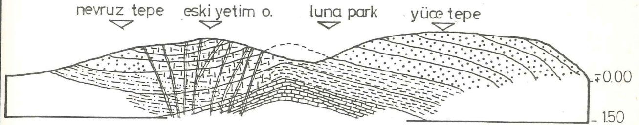
I-I kesiti
