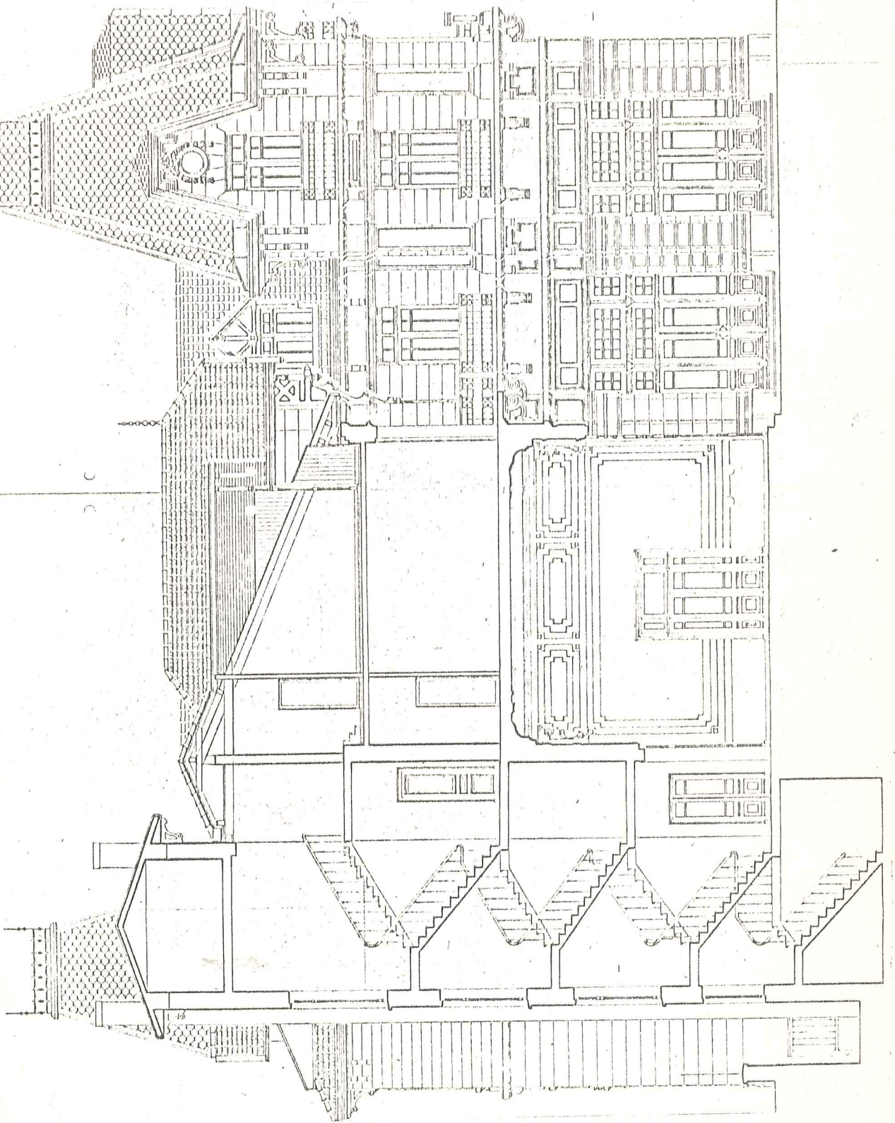
RESİM 30- Anadolu Kulübü, Otel Binası A-A Kesiti
