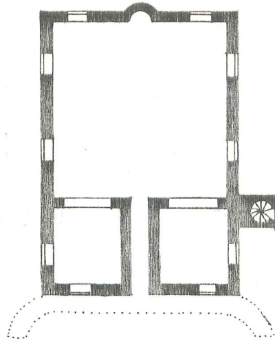
RESİM 20- Büyükada Hamidiye Cami Zemin Kat Planı
